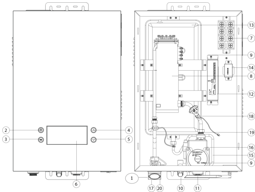
Рис. 1. Конструкция изделия
