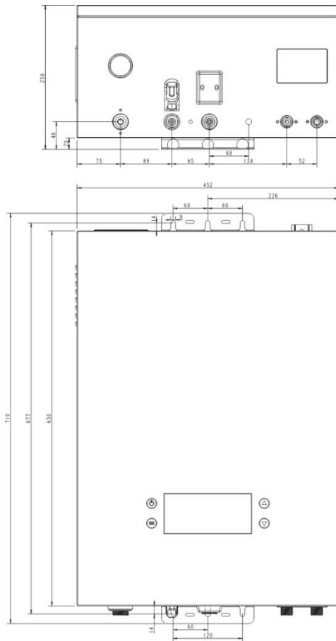
Рис.2. Габаритные размеры
