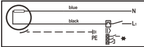
Схема подключения однофазной версии нанесена на табличке электродвигателя
